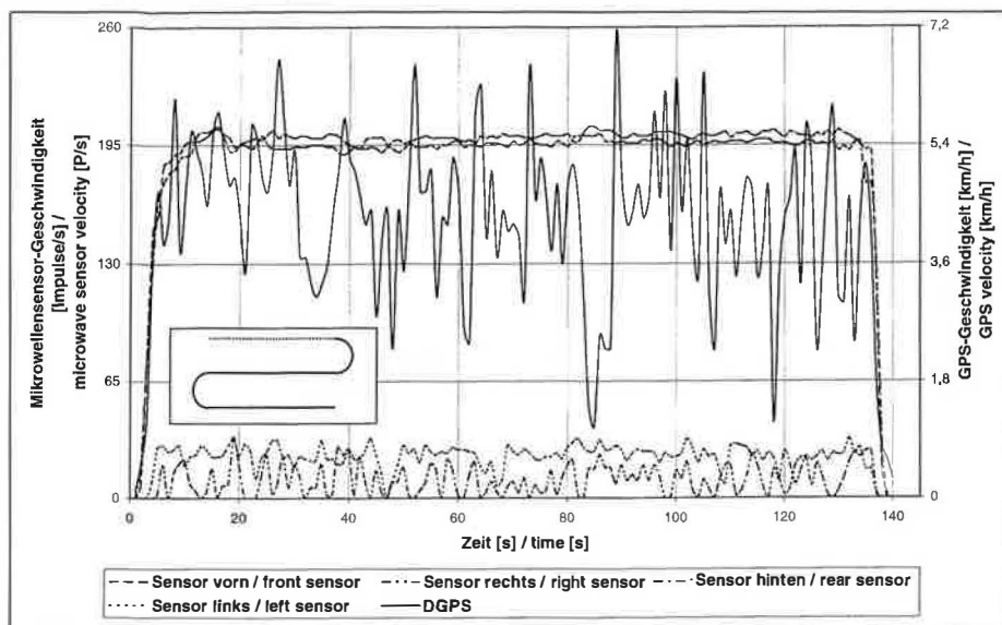
Bild 3: GPS- und Mikrowellensensor-Geschwindigkeit bei Messfahrt in Fahrspur 1 am Waldrand
