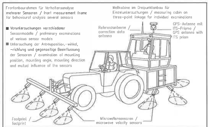
Bild 2: Traktor mit Frontanbau und Messkabine
