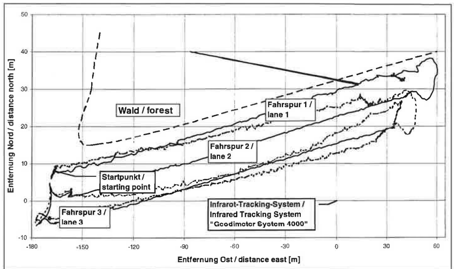
Bild 1: GPS-Abschattung am Waldrand
