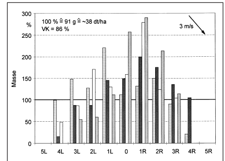
Bild 3: Ungenügende Querverteilung bei 6,10 m Arbeitsbreite (11 Messpunkte mit 0 als Mähdreschermittle, 4 Wiederholungen)
