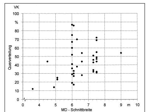
Bild 4: Querverteilung in Abhängigkeit von der Schnittbreite der Mähdrescher
