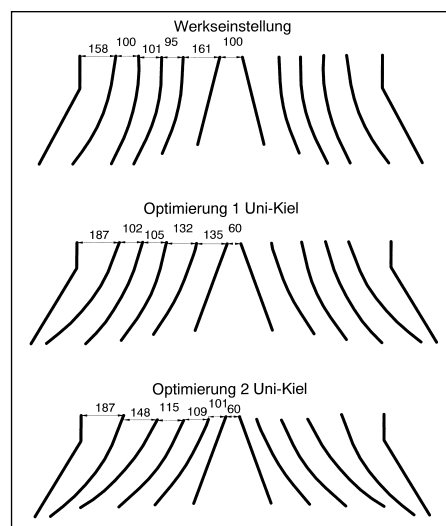
Bild 5: Eingangsabstände (mm) zwischen den Leitblechen häckslerseitig bei einem Mährescher mit 6,30 m Arbeitsbreite (Voßhenrich, Musfeldt, Lubkowitz)
