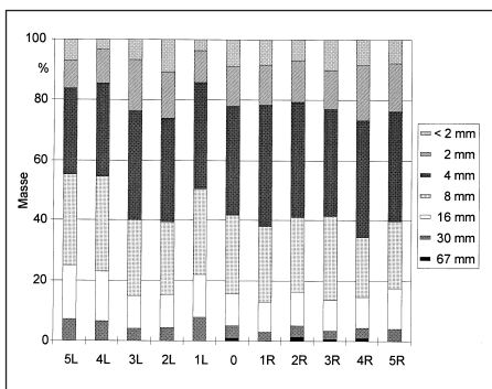
Bild 7: Siebfractionen einer Untersuchung (Rundlochsieb: 2 bis 67 mm Lochdurchmesser)
